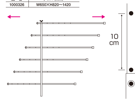
タペストリーポール type L
